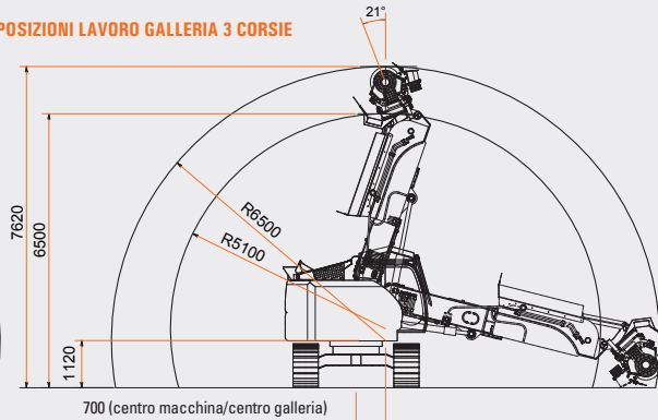
CORSA SFILLO E ROTAZIONE FRESE
